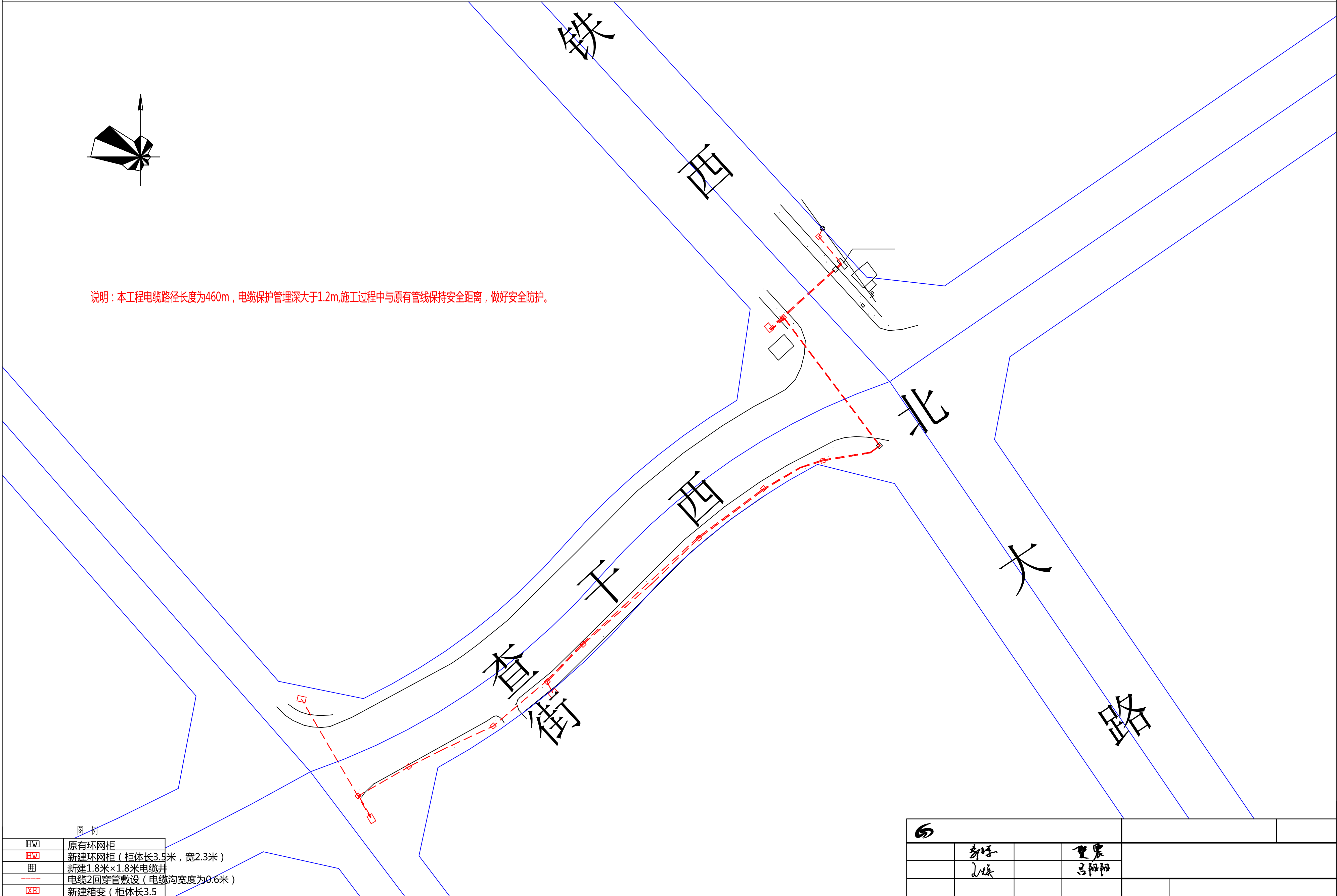
蒙东兴安乌兰浩特供电服务中心2026年城网工程—蒙东兴安城区2026年非直供小区专项第一批0.4kV业扩配套工程等工程—国网蒙东兴安乌兰浩特供电服务中心10kV桥南线万象名邸业扩配套工程总平面布置图
